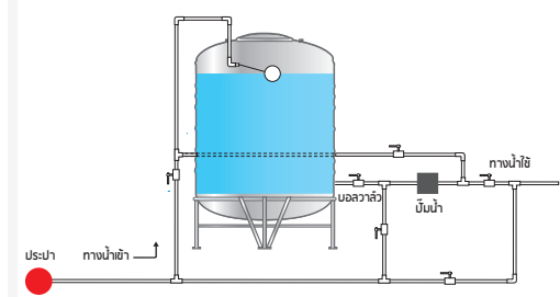
การติดตั้งประปา 4 ระบบ
