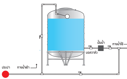
การติดตั้งประปา 2 ระบบ
