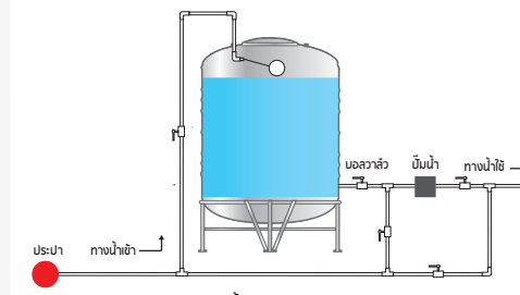
การติดตั้งประปา 3 ระบบ
